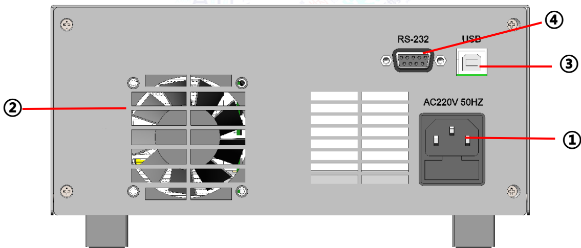
图 2.3.1 设备后面板
