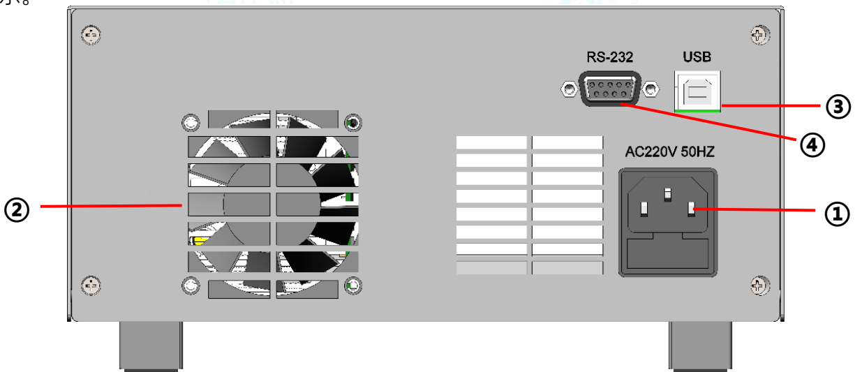
图 2.3.1 设备后面板
