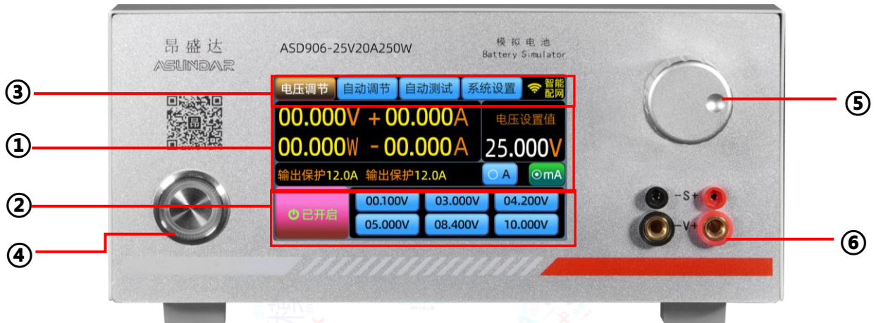
图 2.2.1 设备前面板
