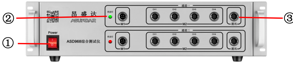
图2.2ASD968前面板
