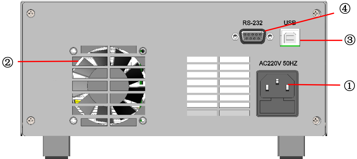
图 2.3.1 设备后面板
