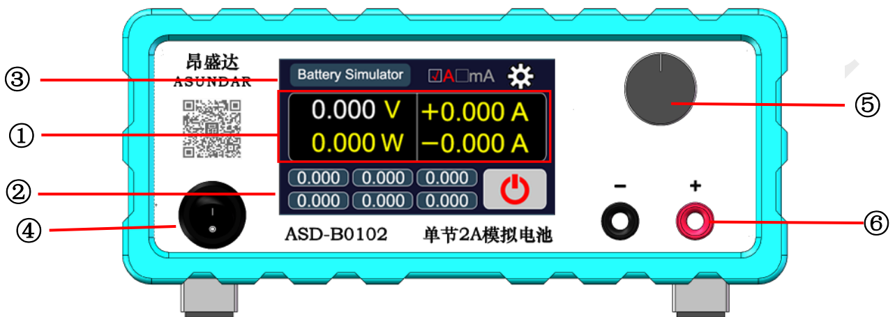
图 2.2.1 设备前面板
