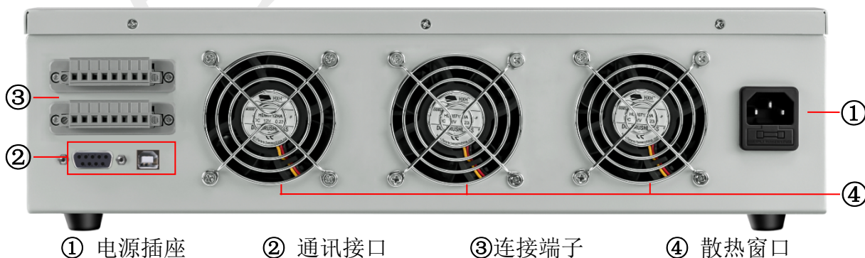
图 6.2.1 测试仪后面板
