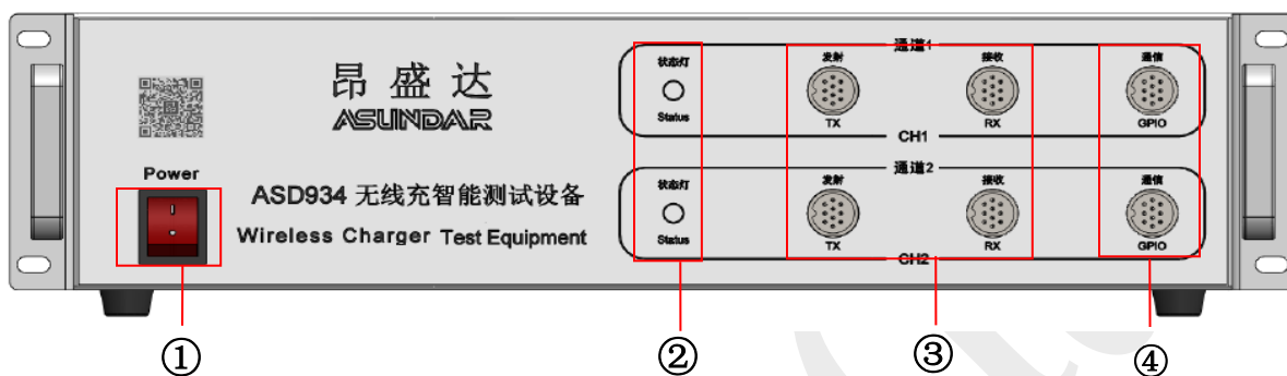
① 电源按钮 ② 状态灯 ③测试接口 ④ 通讯接口
