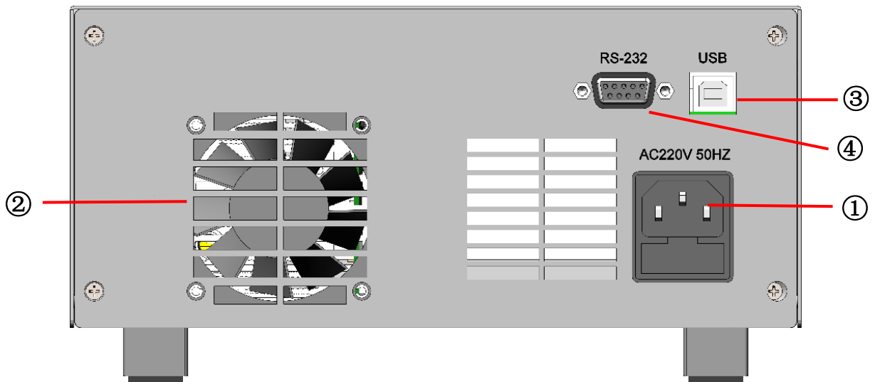
图 2.3.1 设备后面板
