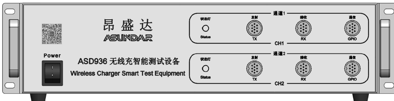
图 2.2: ASD936 前面板
