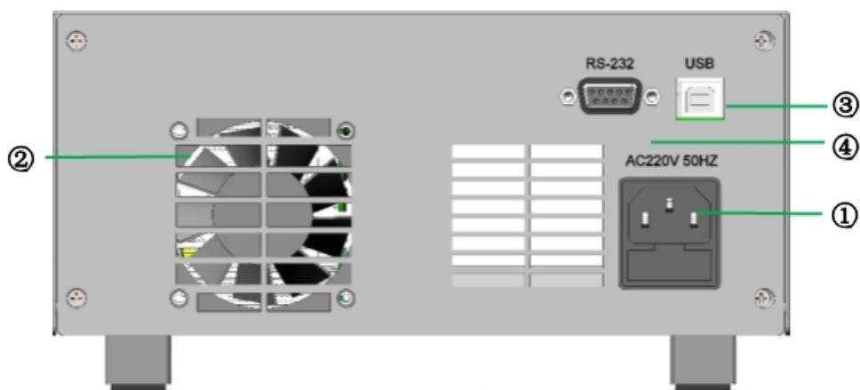
图 2.3.1 设备后面板
