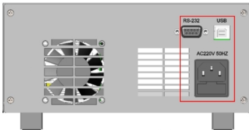
图 6.2.1 模拟电池后面板
