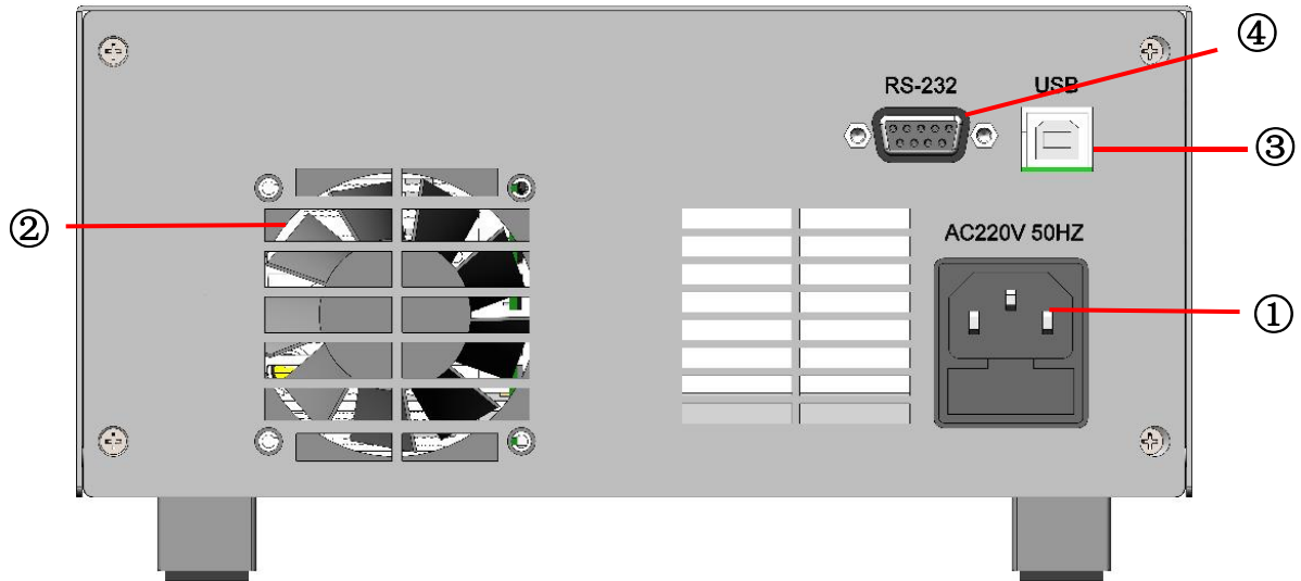
图 2.3.1 设备后面板
