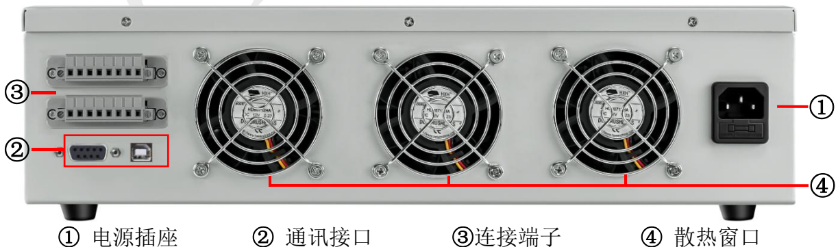
图 6.2.1 测试仪后面板
