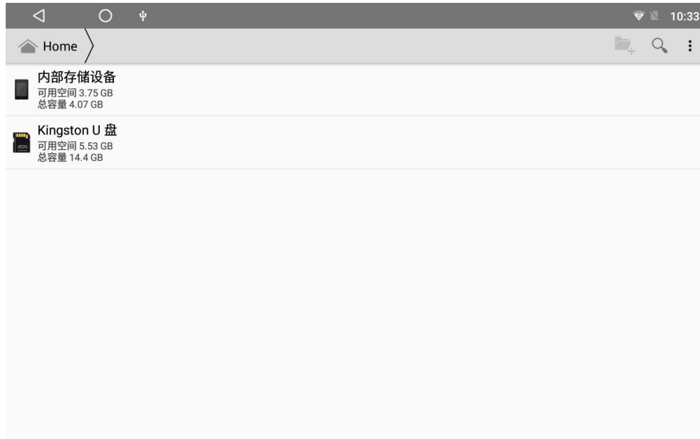
图5.4.3 文件管理器
