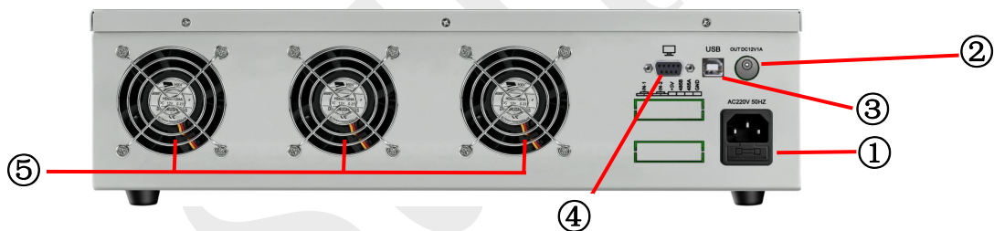
图2.3ASD968A后面板
