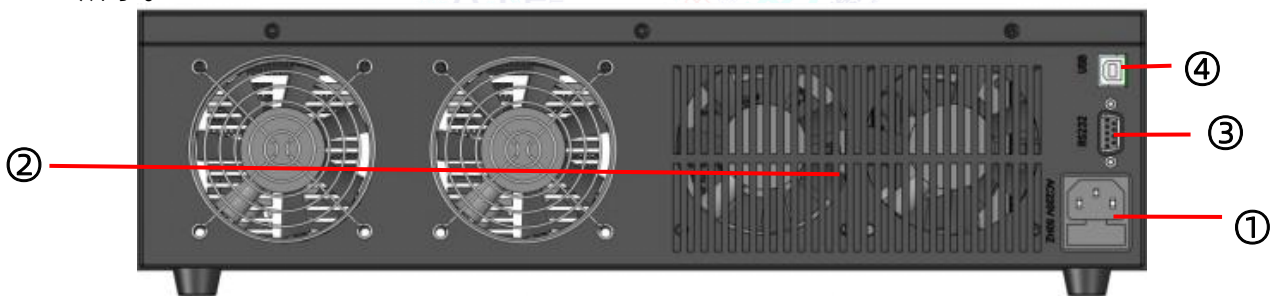
图 2.3.1 设备后面板
